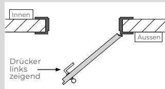
DIN rechts auswärts öffnend
