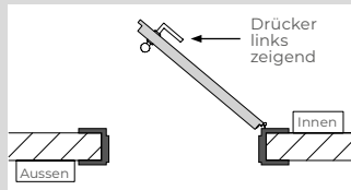
DIN links einwärts öffnend
