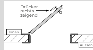
DIN rechts einwärts öffnend
