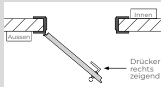
DIN links auswärts öffnend
