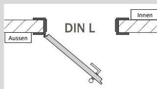
links auswärts öffnend
