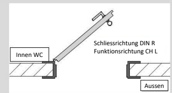
Türe rechts einwärts öffnend
