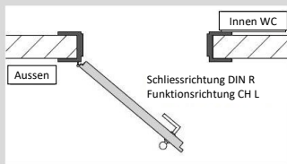
Türe links auswärts öffnend
