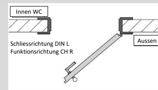
Türe rechts auswärts öffnend
