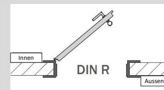
rechts einwärts öffnend
