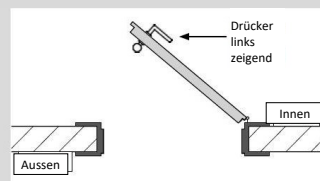
DIN links einwärts öffnend
