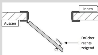
DIN links auswärts öffnend
